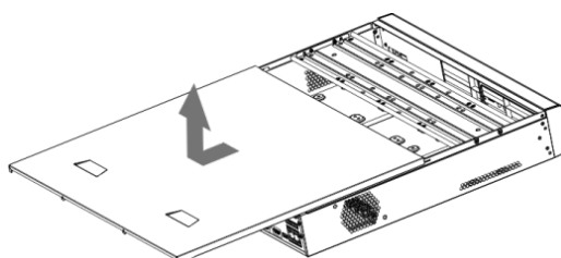
Figure 2-17 Retire la cubierta
