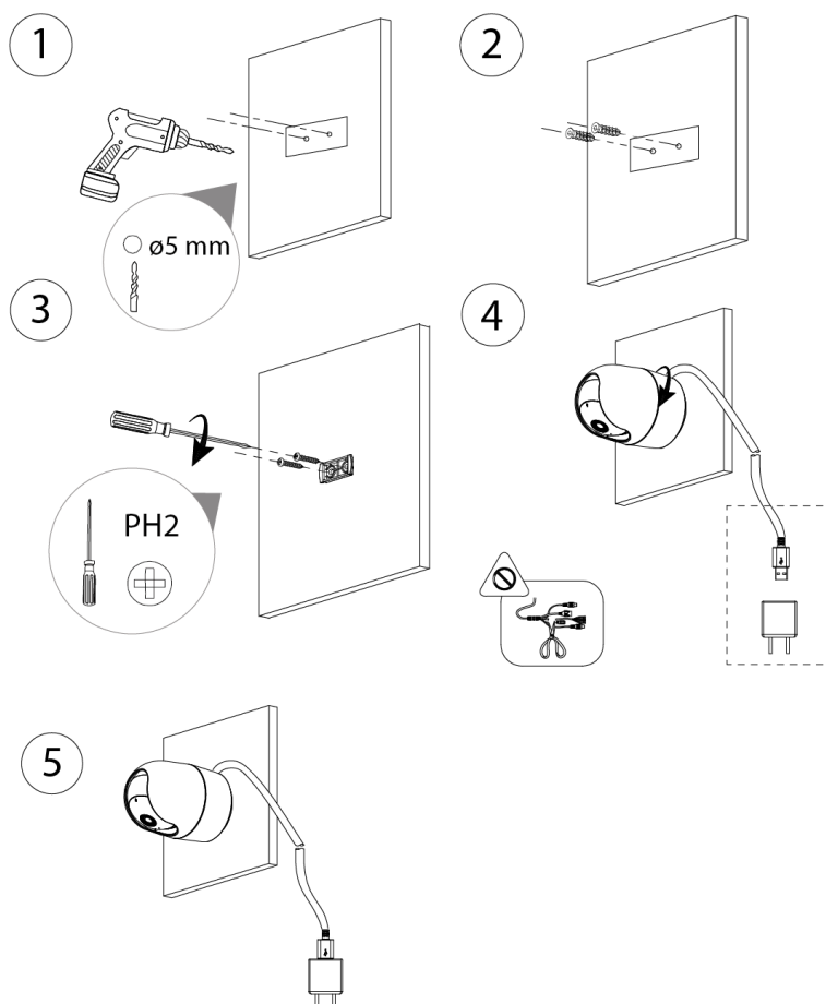
Figura 3-3 Colocación de la cámara
