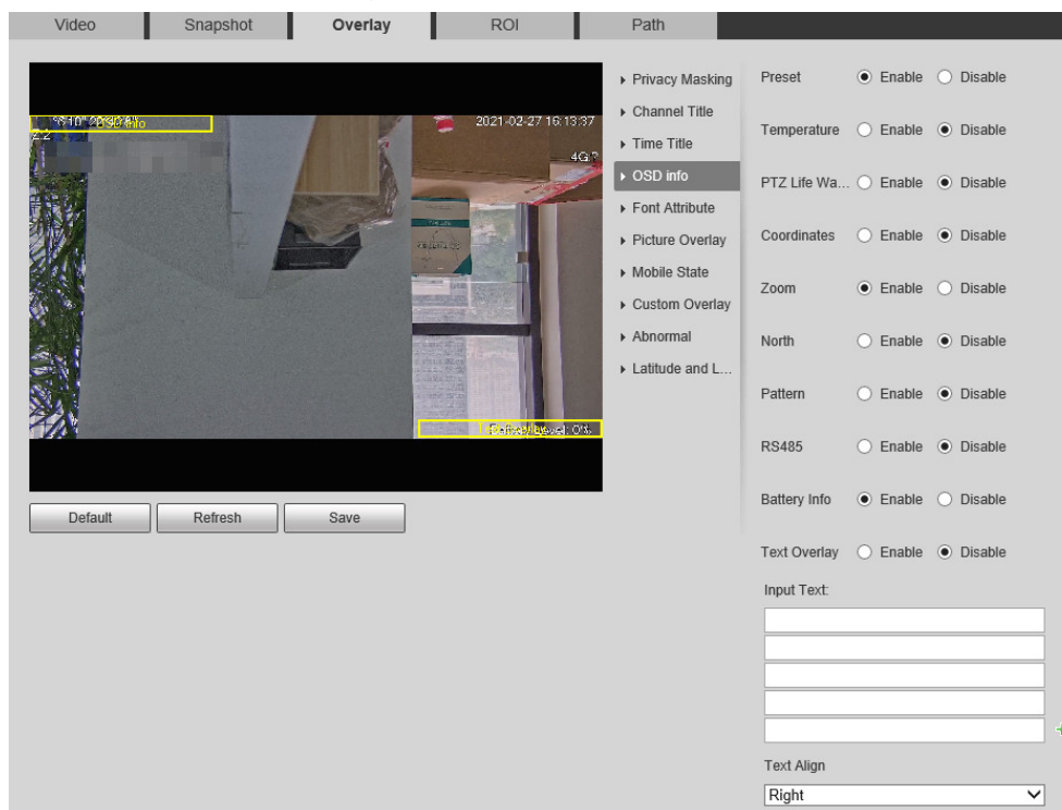
Figura 5-23 Información OSD
