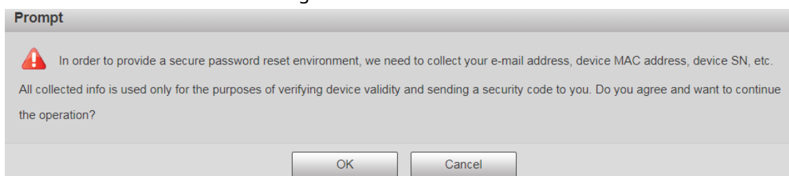
Figura 1-15 Aviso
