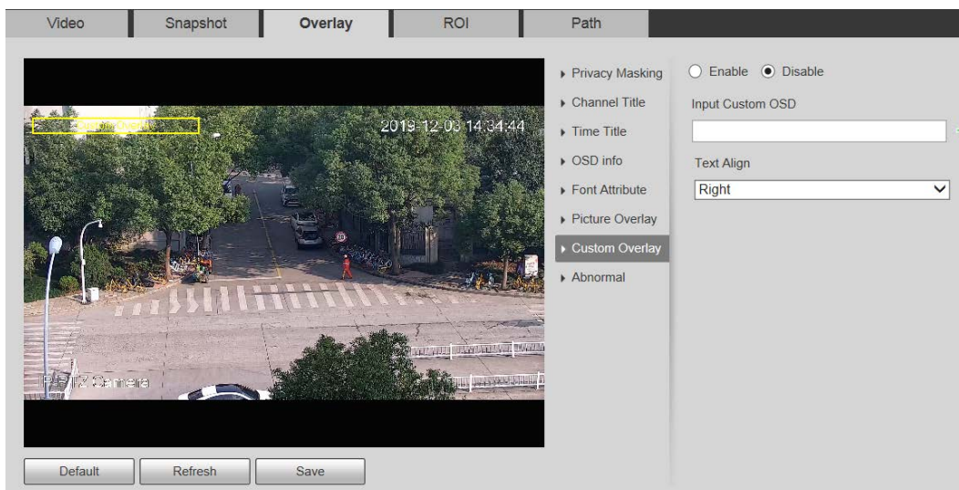
Figura 5-27 Superposición personalizada
