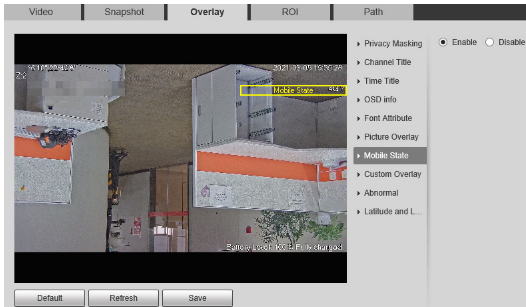
Figura 5-26 Estado móvil
