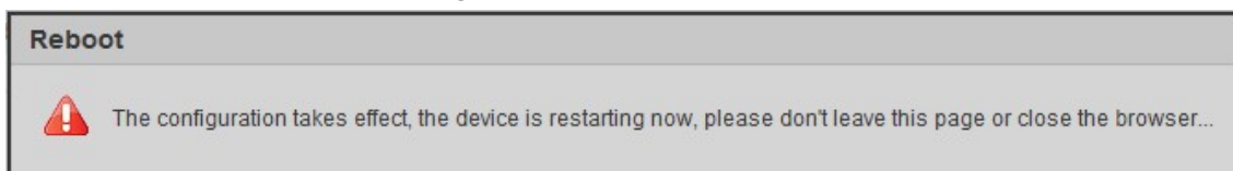
Figura 5-171 Reiniciar
