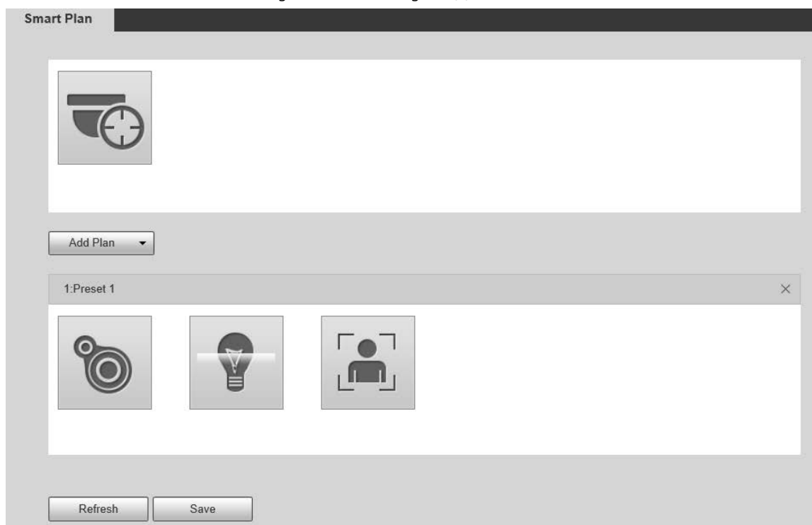
Figura 5-88 Plan inteligente (1)
