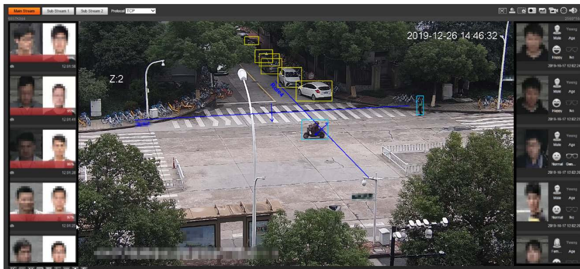
Figura 2-8 Cara
