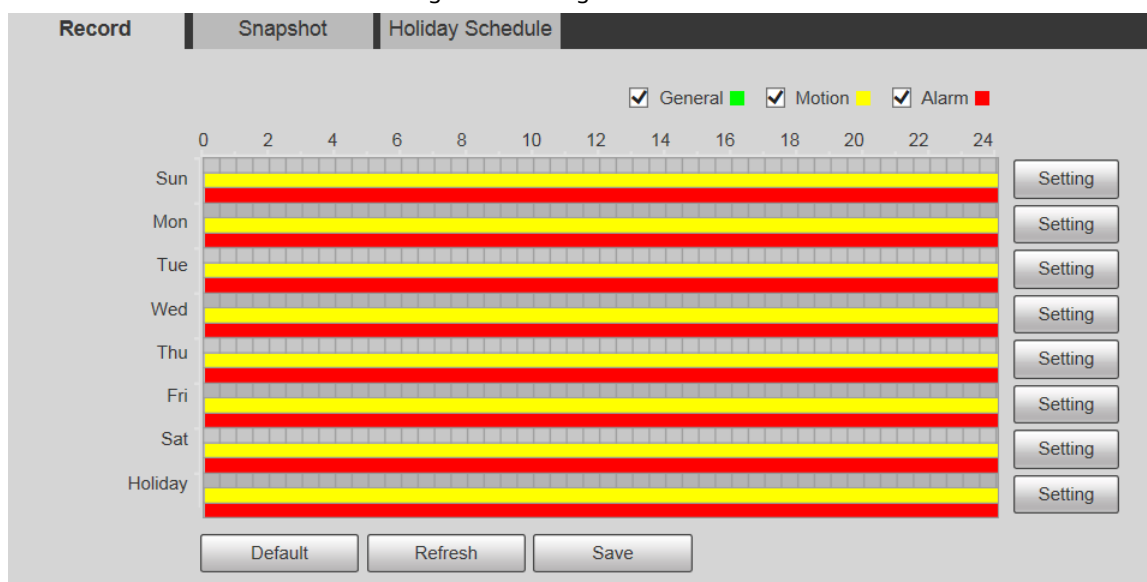
Figura 5-134 Registro
