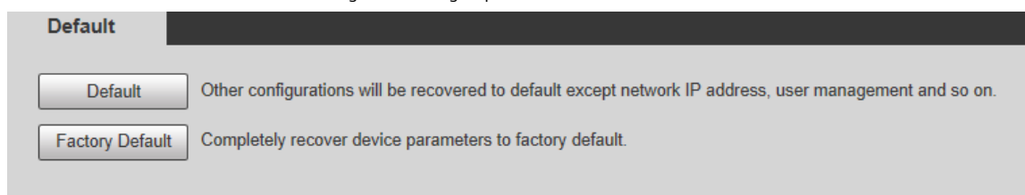
Figura 5-174 Página predeterminada
