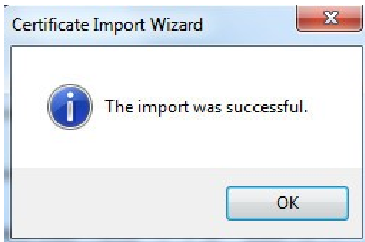
Figura 5-169 Importación exitosa
