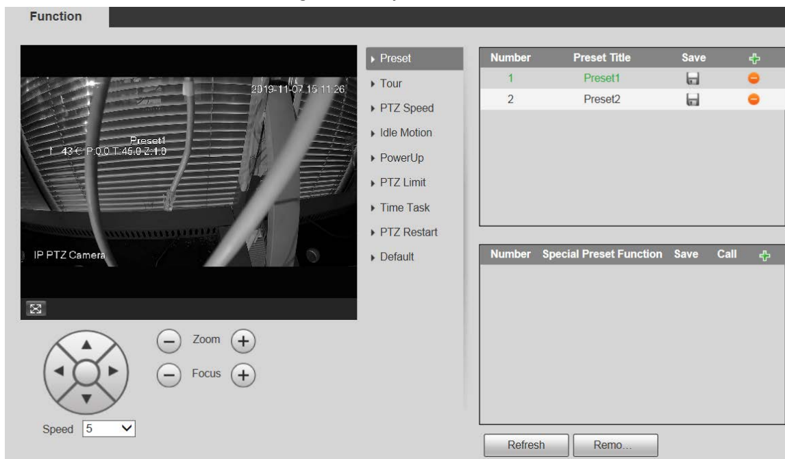
Figura 5-67 Preajuste
