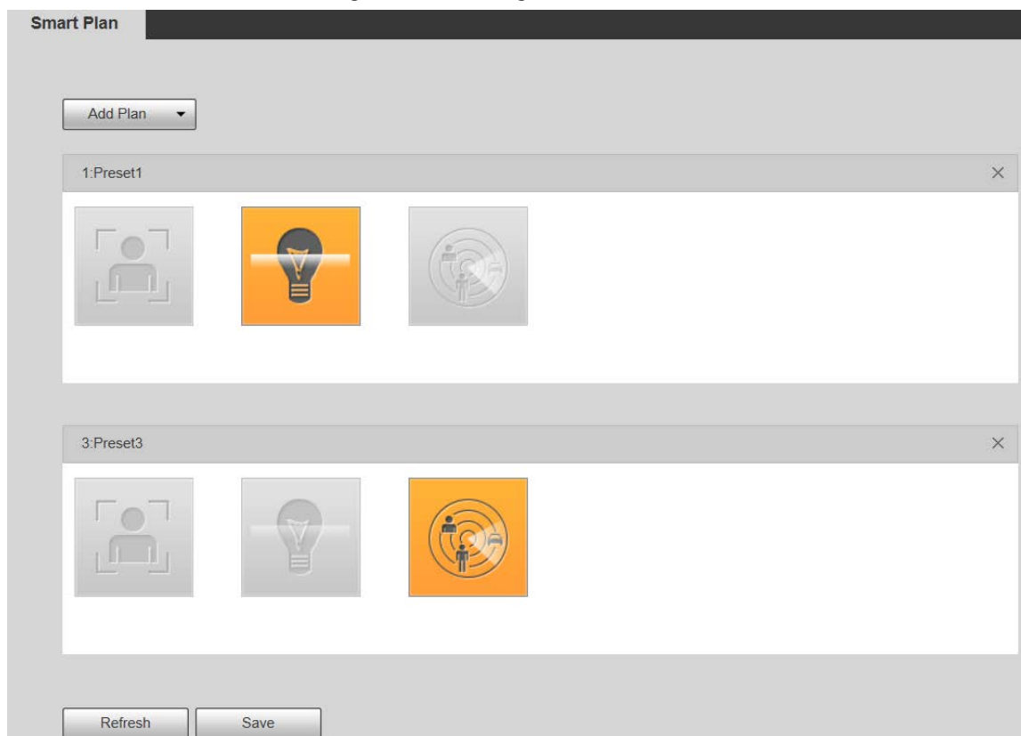
Figura 5-89 Plan inteligente (2)
