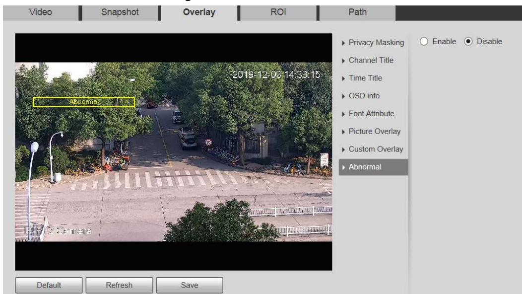
Figura 5-28 Anormal
