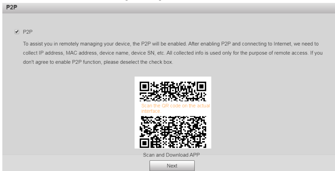
Figura 1-8 Página P2P
