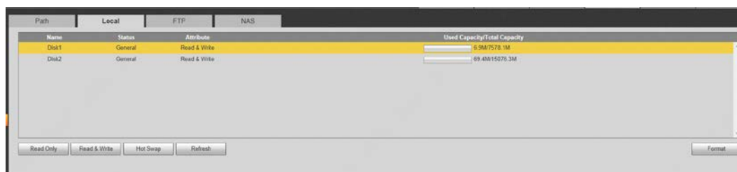
Figura 5-142 Almacenamiento local
