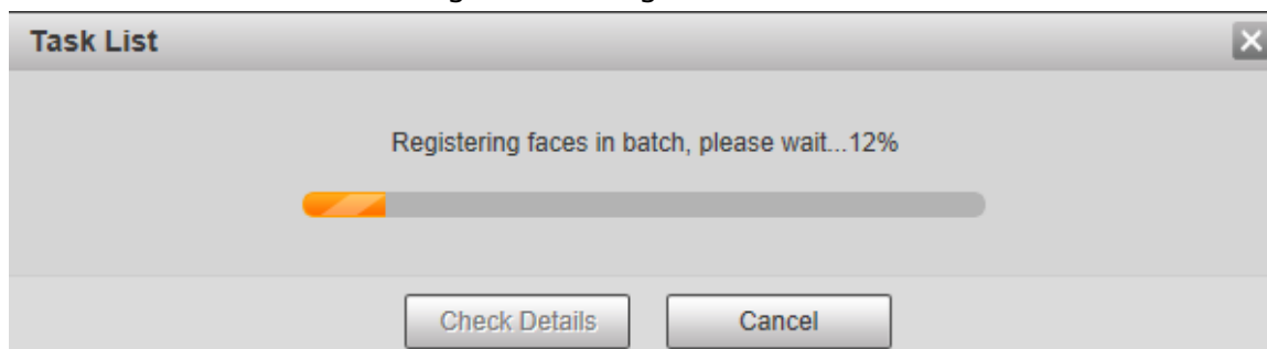
Figura 5-111 Registro
