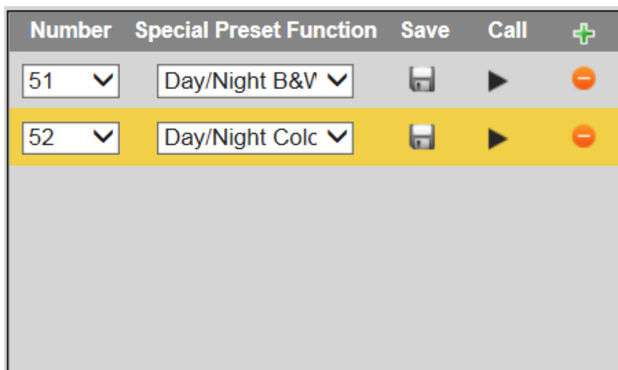
Figura 5-69 Preajustes especiales
