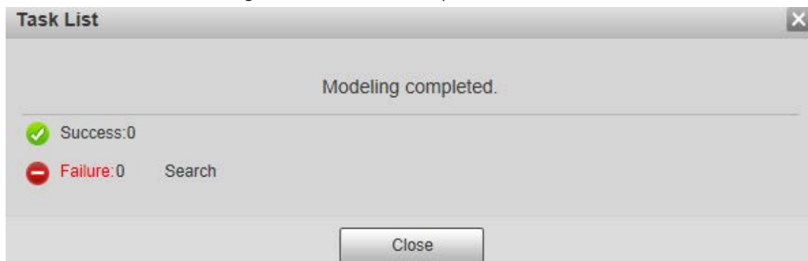
Figura 5-114 Modelado completado
