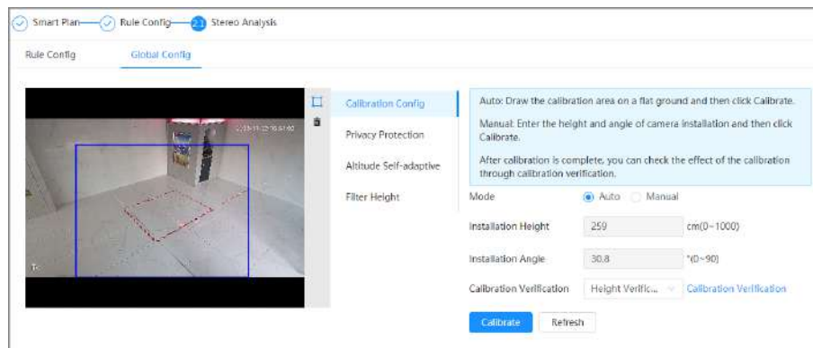
Figura 8-77 Configuración global del análisis estéreo
