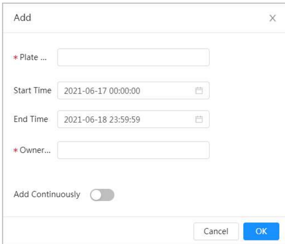
Figura 8-66 Agregar placa de lista de permitidos
