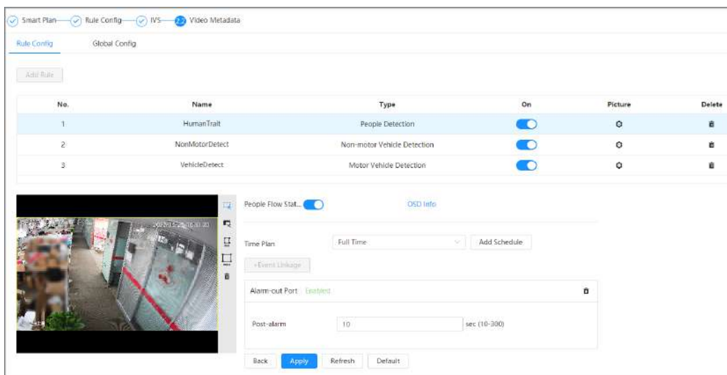
Figura 8-76 Establecer metadatos de video
