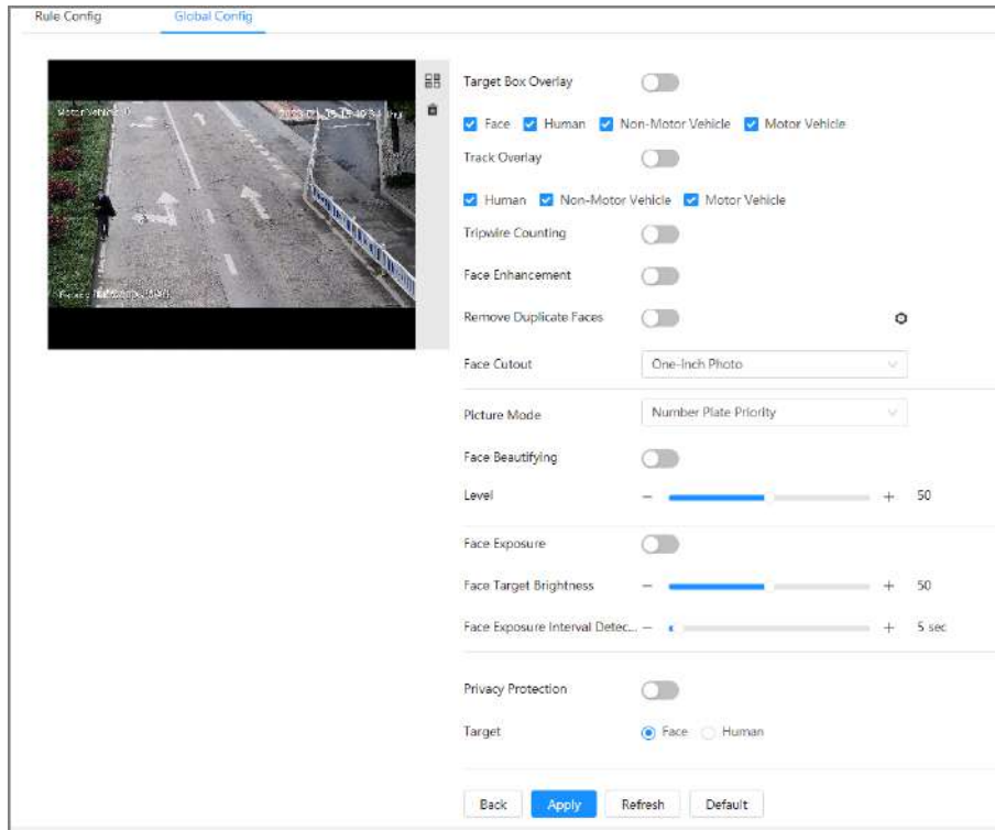
Figura 8-40 Configuración global de metadatos de video (2)
