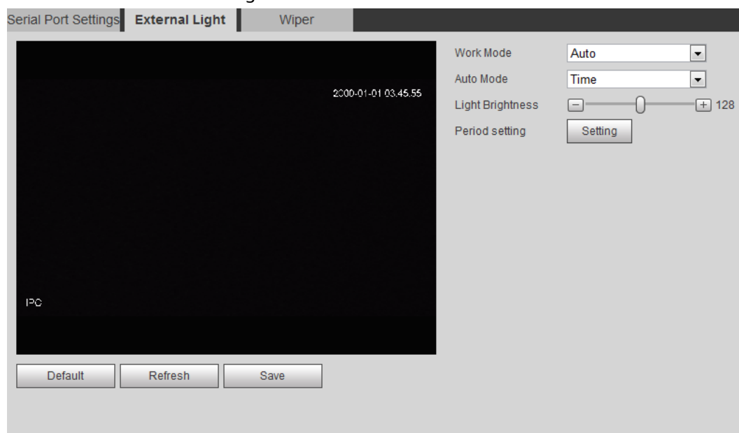
Figura 4-122 Luz exterior
