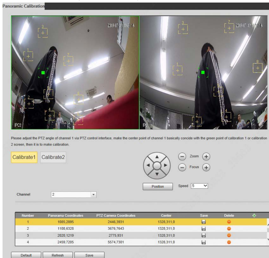
Figura 5-20 Calibración panorámica
