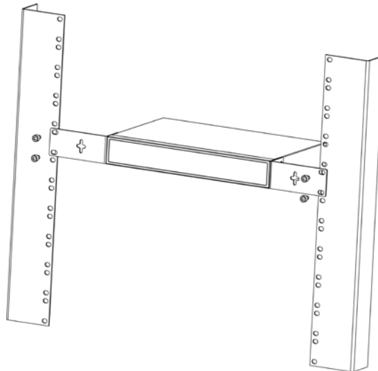
Figura 3-2 Fije el interruptor en el bastidor
