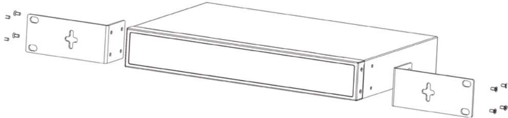
Figura 3-1 Coloque los soportes de montaje
