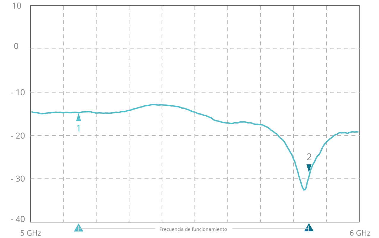
Pérdida de retorno – Polarización vertical
